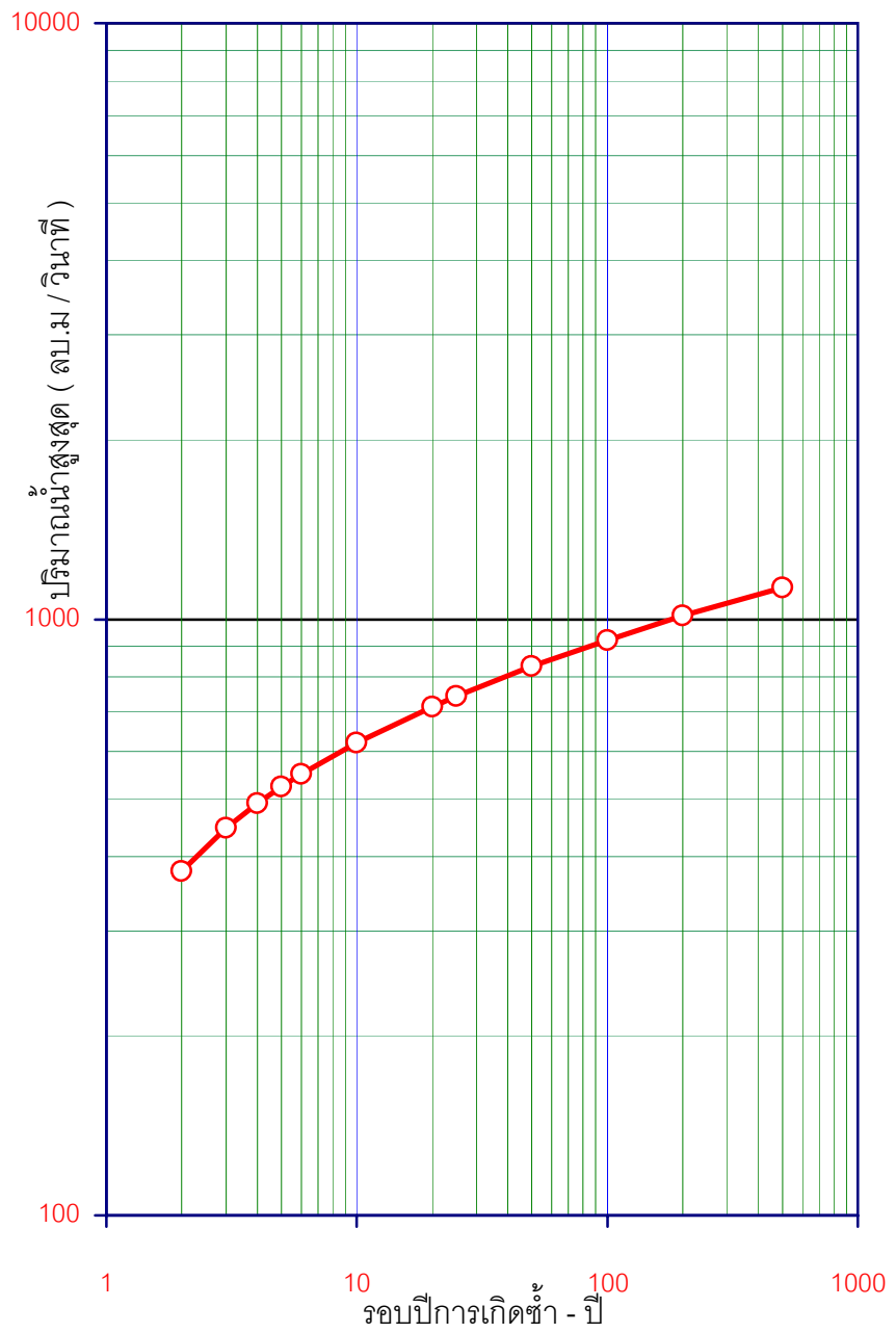
ปริมาณน้ำสูงสุดรายปี-ลบม./วินาที สถานี P.1 แม่น้ำปิง อ.เมือง จ.เชียงใหม่
