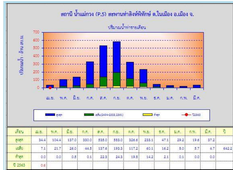
กราฟแสดงปริมาณน้ำทำรายเดือนสถานี Sw.5A น้ำปาย บ้านท่าโป่งแดง อ.เมือง จ.แม่ฮ่องสอน
