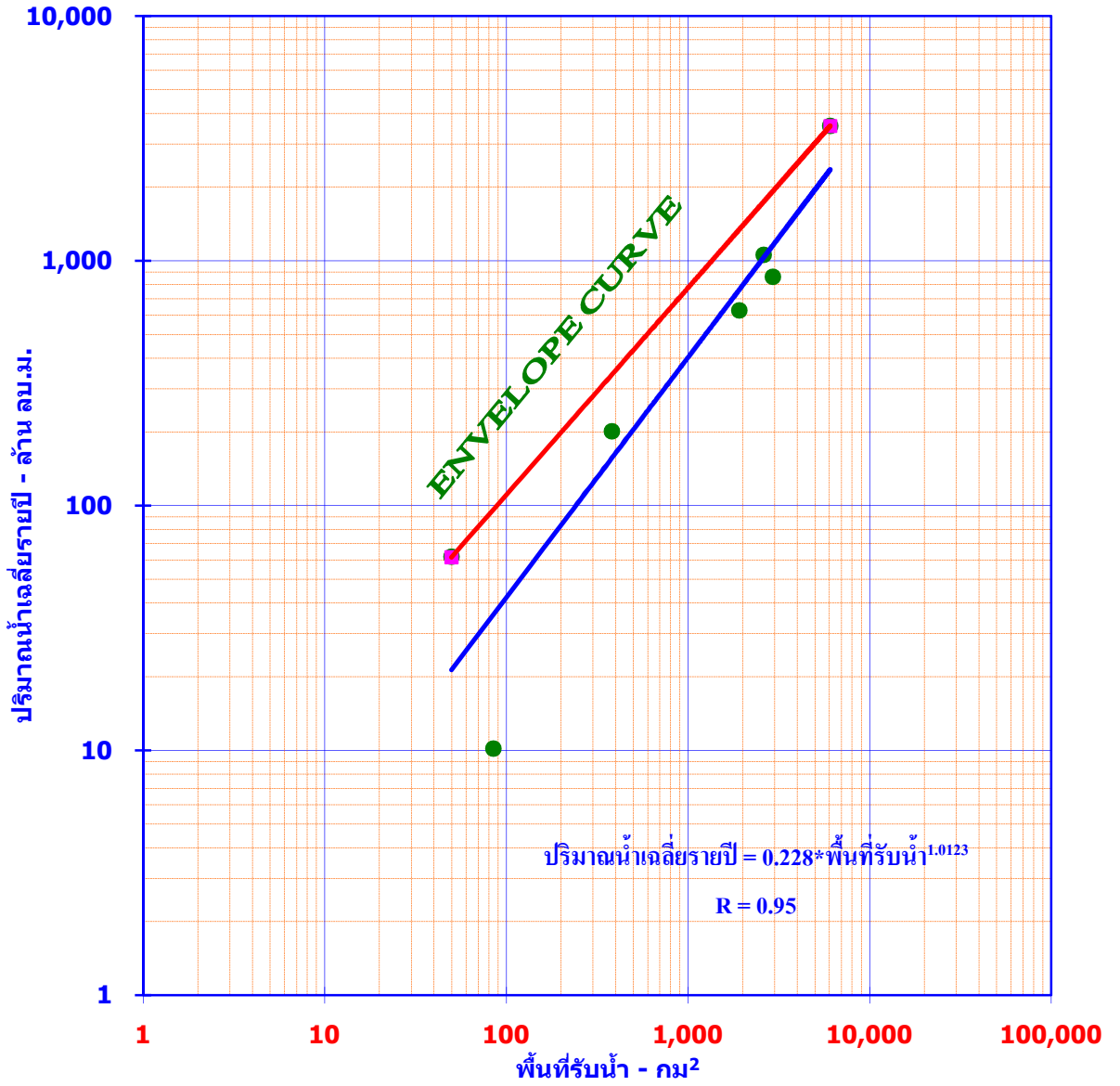
ความสัมพันธ์ระหว่างปริมาณน้ำเฉลี่ยรายปีและพื้นที่รับน้ำของลุ่มน้ำกก
