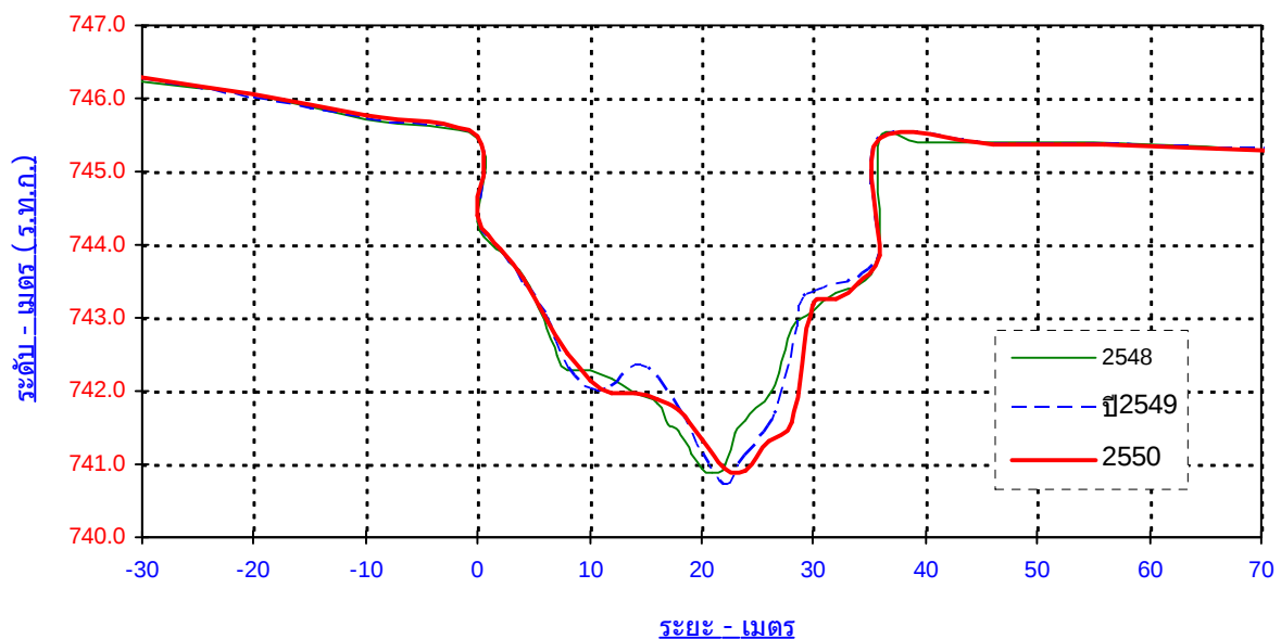
รูปตัดขวางน้ำแม่แดง สถานี P.65 อ.เวียงแหง จ.เชียงใหม่
