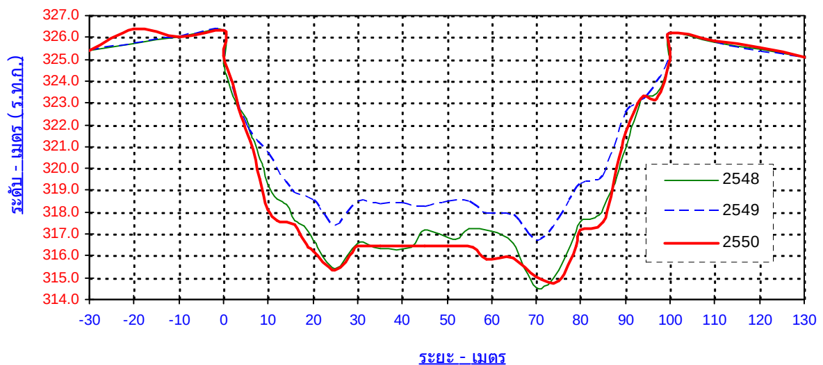
รูปตัดขวางแม่น้ำปิง สถานี P.67 อ.สันทราย จ.เชียงใหม่
